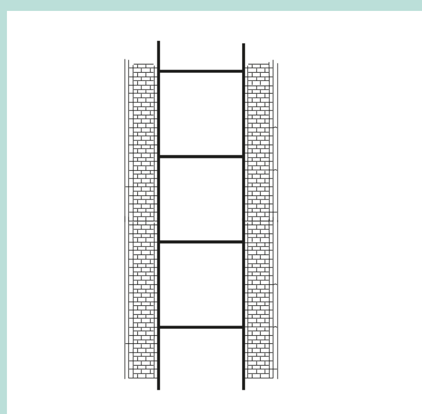
OPBOUW HEMBRUGS STRAATPROFIEL
